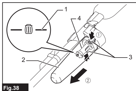
Fig.38 ► 1. Línea de llenado completo 2. Caja para polvo 3. Botón (dos ubicaciones) 4. Filtro de malla
