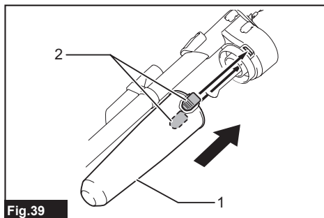
Fig.39 ► 1. Caja para polvo 2. Botón (dos ubicaciones)
